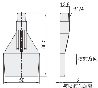
标准型·平行式喷射(铝合金) NHR72
