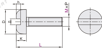
一字槽盘头螺钉 BOX-TAP25
