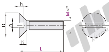
一字槽沉头螺钉 BOX-TAP21
