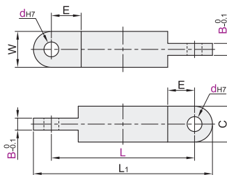
圆耳板型 ZFL14/15/16
