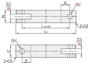
方耳板型 ZFL21/22/23
