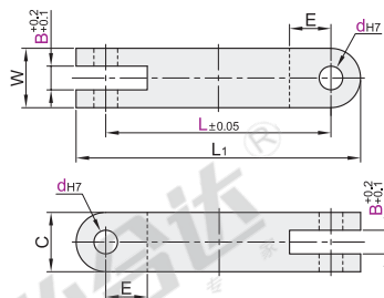
圆耳板型 ZFL24/25/26
