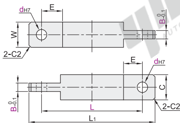
方耳板型 ZFL11/12/13
