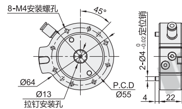
法兰型 ZFH54 带传感器
