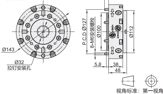
法兰型 ZFH54 带传感器
