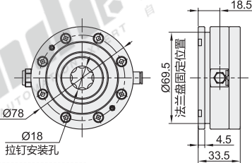
台面型 ZFH52 无传感器
