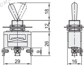
双极双投型 ZHB86-2-2
