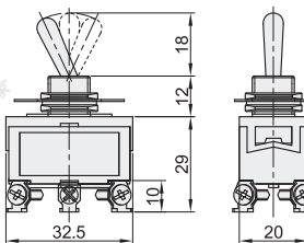
双极双投中间停型 ZHB86-2-3
