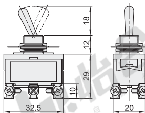
双极双投型 ZHB86-2-2
