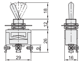
双极双投中间停型 ZHB86-2-3
