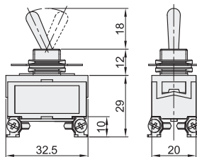
双极单投型 ZHB86-2-1
