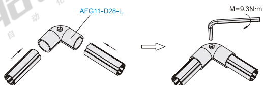
分解图
