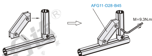
分解图
