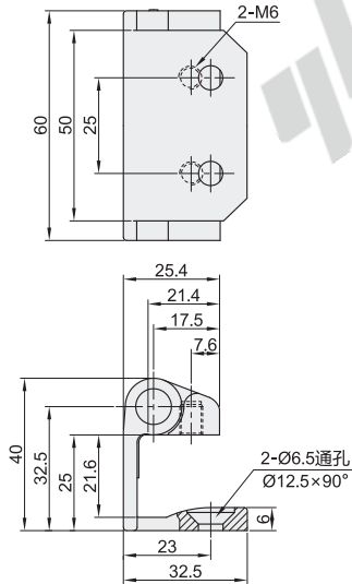
安装图
