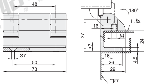
HFS25(锥孔+螺孔型)
