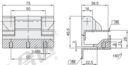
HFS26(螺孔型)
