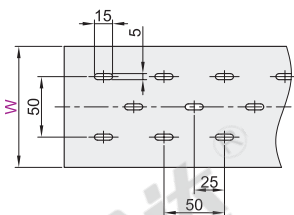
W≥80mm线槽底部孔尺寸
