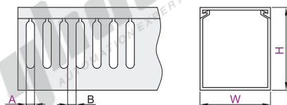
W≤60mm线槽底部孔尺寸
