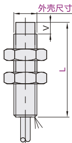
非齐平式 ZJG41 外壳尺寸:M8
