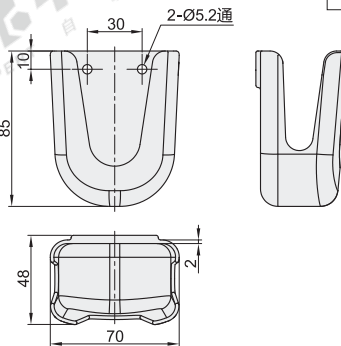
椭圆形 ZCQ02
