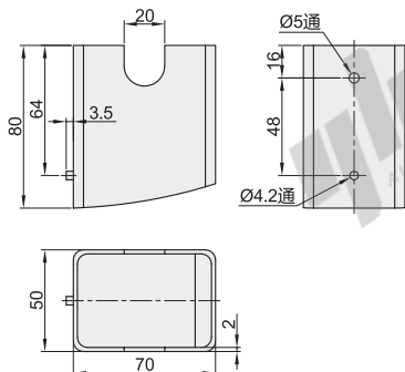
方形 ZCQ01
