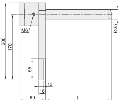
挂料架
