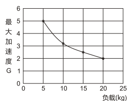
最大加速度VS负载
