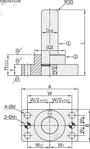
自润滑型-带定位孔型 OFQ34
