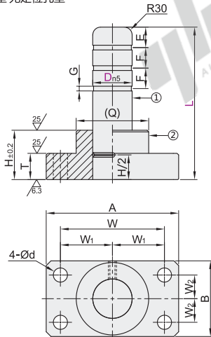
油润滑型-无定位孔型 OFQ31
