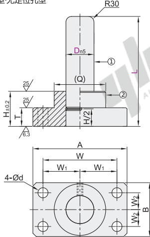
自润滑型-无定位孔型 OFQ33
