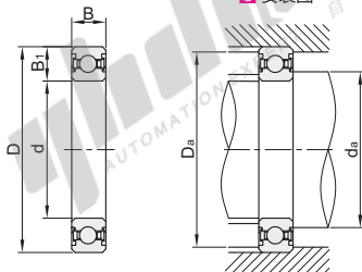
安装图
