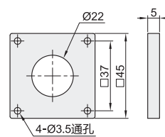
法兰尺寸
