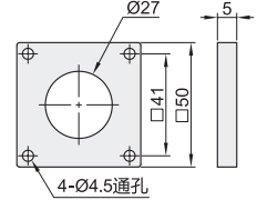
法兰尺寸
