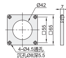
法兰尺寸
