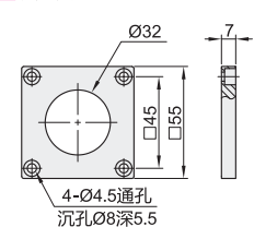
法兰尺寸
