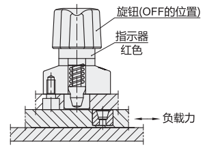
旋钮在OFF的状态
