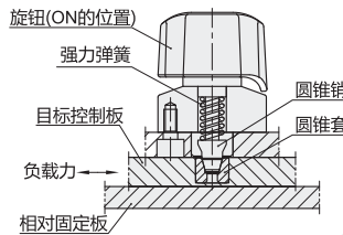
旋钮在ON的状态
