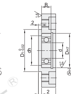
引导型·带挡圈型 BFT03
