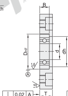
标准型·无挡圈型 BFT01
