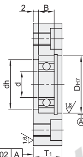
标准型·带挡圈型 BFT02
