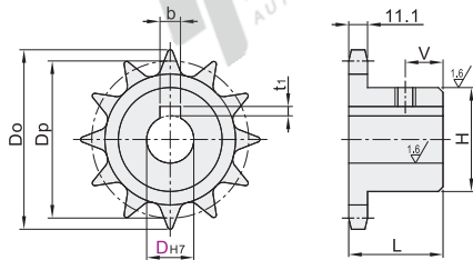
链轮 VLY31/32
