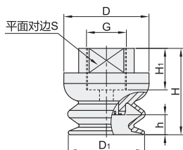
内接螺纹 外形A
