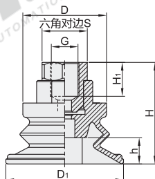
内接螺纹 外形B
