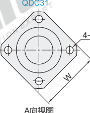
方法兰式 QDC31
