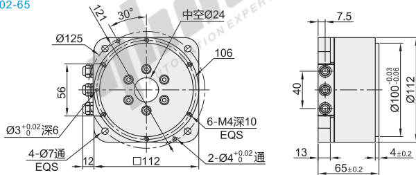
电机高度：65 ZJC02-65
