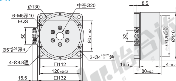
电机高度：80 ZJC03-80
