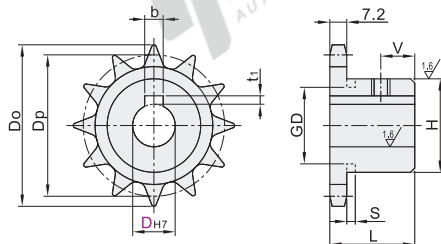
链轮 VLY11/12
