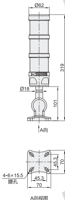
A向视图
