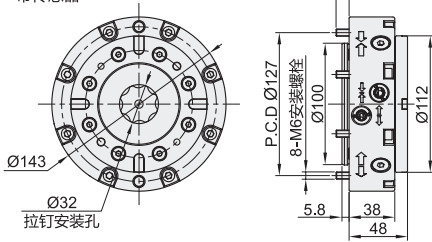
法兰型 ZFH54 带传感器
