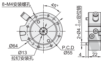
法兰型 ZFH54 带传感器
