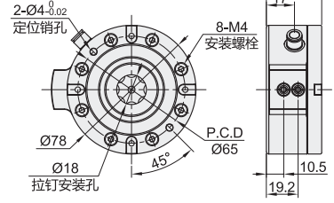
台面型 ZFH53 带传感器
