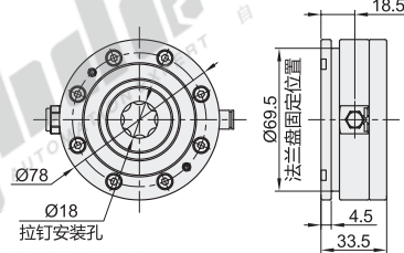
台面型 ZFH52 无传感器
