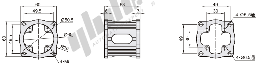
■ M3(80法兰伺服电机座、86法兰步进电机座)
