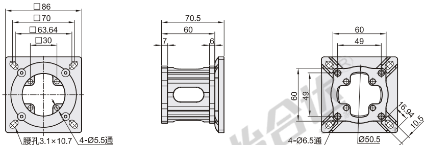
■ M3(80法兰伺服电机座、86法兰步进电机座)
