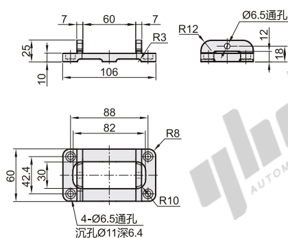
■ M1(57法兰步进电机座)
