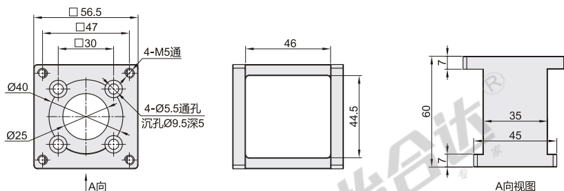
■ M2(60法兰伺服电机座)
