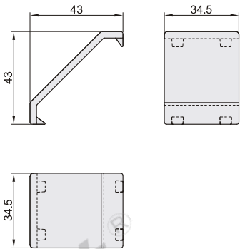
盖板 (配套使用)
