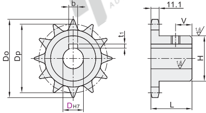
链轮 VLY31/32
