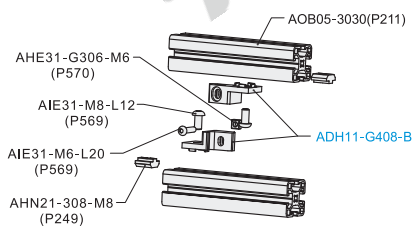
分解图
