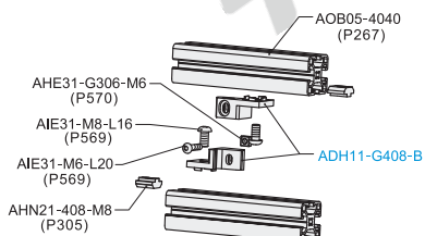
分解图
