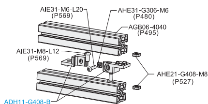
分解图
