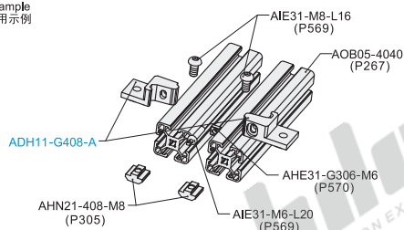
分解图
