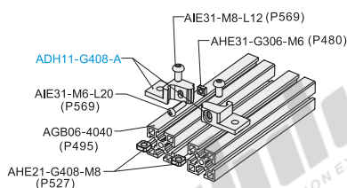
分解图
