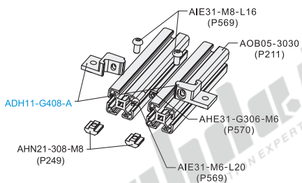
分解图
