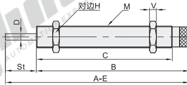
无撞击头 J-WJC01
