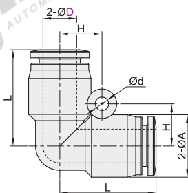
弯接头 XZS22
