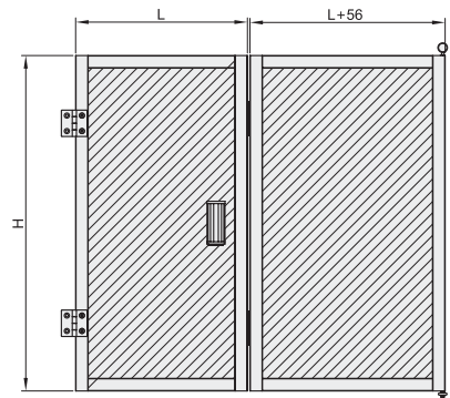
门框开料尺寸
