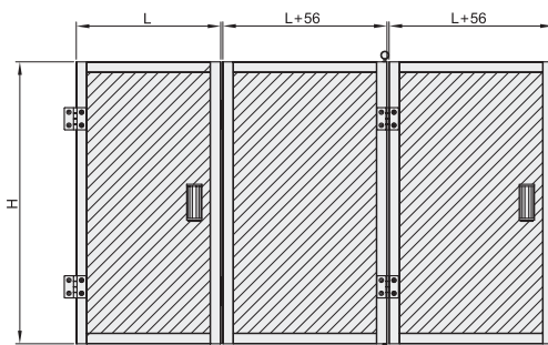
门框开料尺寸
