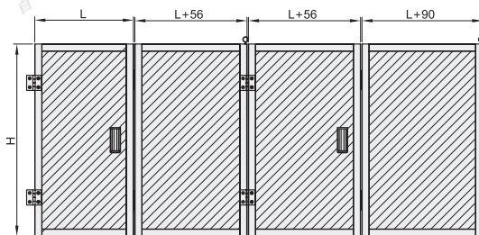
门框开料尺寸
