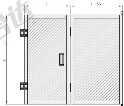
门框开料尺寸
