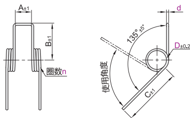
角度135° FHC22
