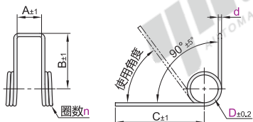
角度90° FHC21
