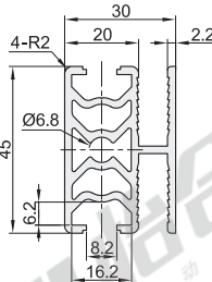
ATS02-H3045W 重量:1.28Kg/m
