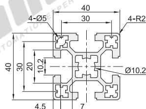
AOB02-H4040E 重量:1.56Kg/m
