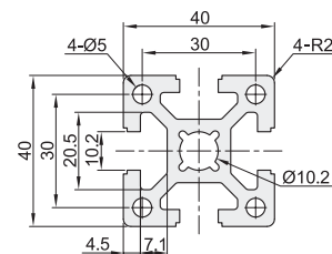
AOB02-H4040 重量:2Kg/m
