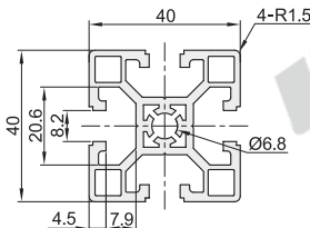
AOB05-4040F 重量:1.48Kg/m
