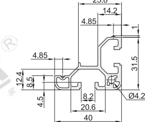
ATS05-3340W 重量:0.69Kg/m
