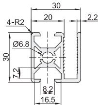
ATS05-3030W 重量:0.84Kg/m
