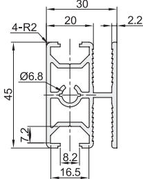
ATS05-3045W 重量:1.12Kg/m
