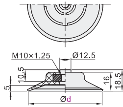
盘径Ø150
