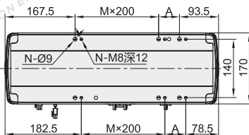
A向视图
