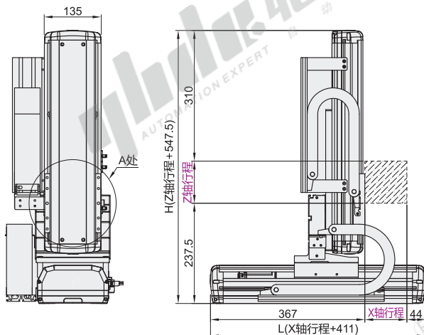
❑ XZ轴拖链
