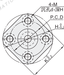
方法兰 BFF61/62/63/64/66
