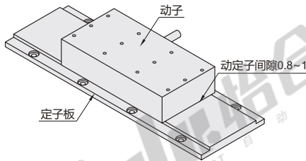
动子与定子板配合示意图
