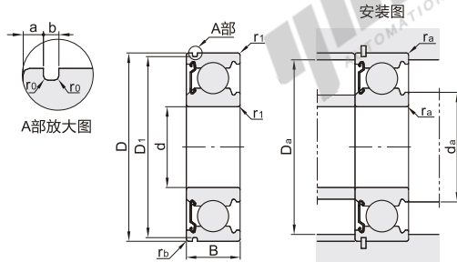
ZN(一面带防尘盖一面带止动槽)
