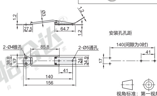
长臂型 HFQ64
