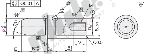
多棱型 YDR31/35
