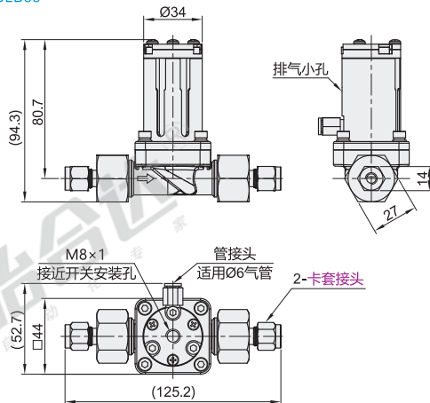
高压型 BLB85
