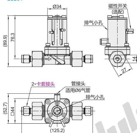
常规型 BLB84
