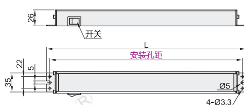
标准型 ZHE75
