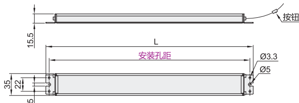
经济型 ZHE30
