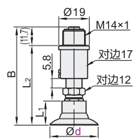
弹簧式直接安装型 J-WET76/77
