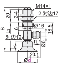
弹簧式侧面真空端口 J-WET71/72
