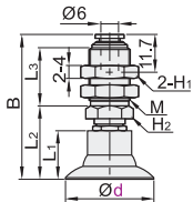
弹簧式侧面真空端口 J-WET71/72
