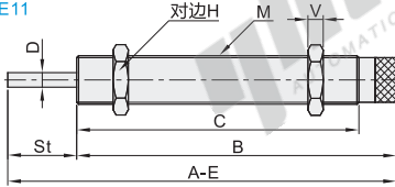
外置复位弹簧 J-WJE01
