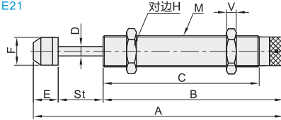
外置复位弹簧 J-WJE01
