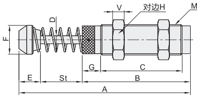
外置复位弹簧 J-WJE01
