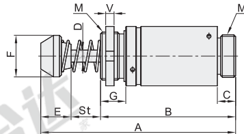
外置复位弹簧 J-WJE01
