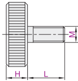
无台阶 外螺纹型 HAW21/22/23/24
