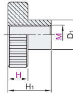
内螺纹型 HAX26/27/28
