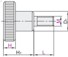
带台阶 外螺纹型 HAW26/27/28/29
