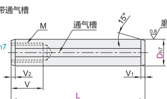
通气槽尺寸图
