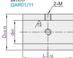
直柱形 QAR01/11
