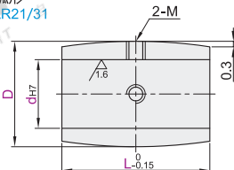
圆弧形 QAR21/31
