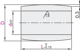
圆弧形 QAQ21/22
