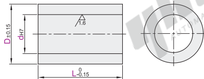
直柱形 QAQ01/02/11/12
