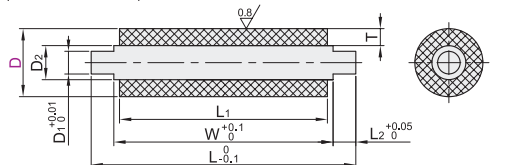
QAA02 (芯材材质: S45C)
