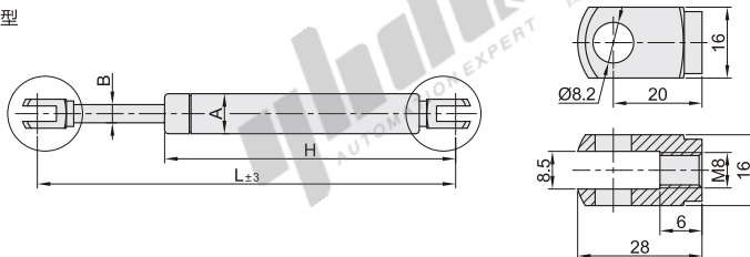
头部安装定向型 FHJ12
