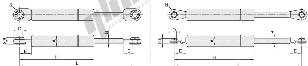
头部安装限定型 FHJ16/E-FH16 规格: 15050A~18100A
