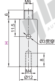
外螺纹型 BMZ27
