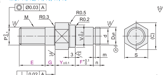
台阶型 MGP11/12/14/16/17/18
