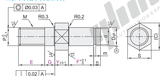
标准型 MGP01/02/04/06/07/08
